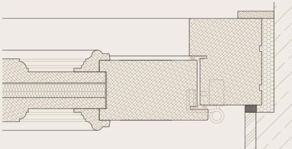
Горизонтальное сечение: коробка, притвор с уплотнением, полотно и стеклопакет в раскладке
