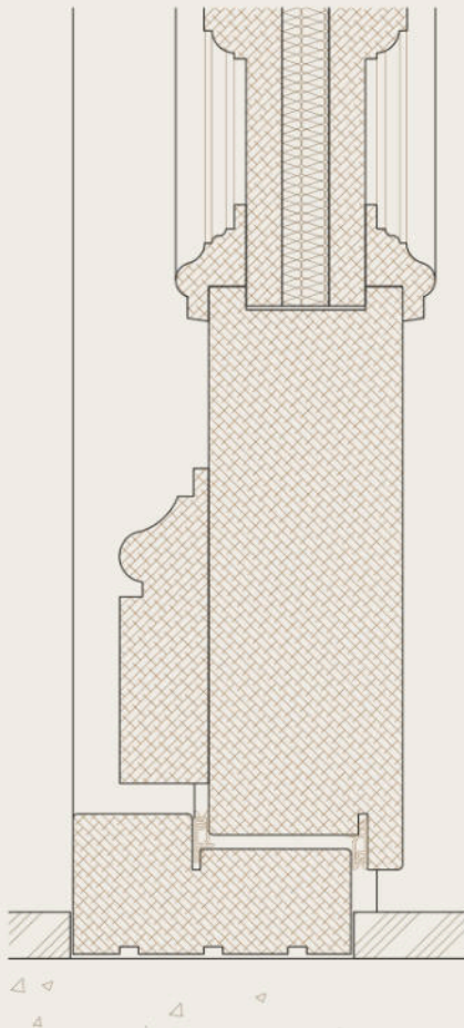
Нижний узел: полотно, порог, примыкание к полу
